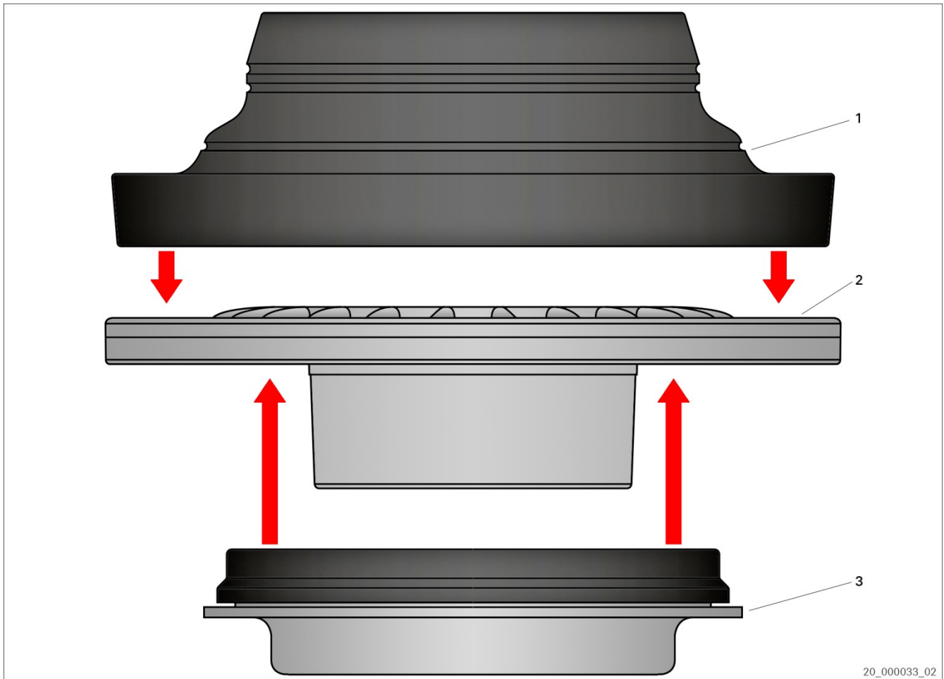
Rys. 1: Montaż łożyska oporowego amortyzatora teleskopowego (przykład)
